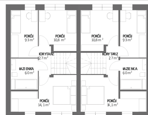
PIĘTRO SEGMENT L+G PIĘTRO SEGMENT P
