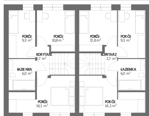
PIĘTRO SEGMENT L PIĘTRO SEGMENT P+G
