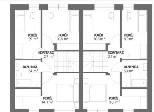
PIĘTRO SEGMENT L+G PIĘTRO SEGMENT P
